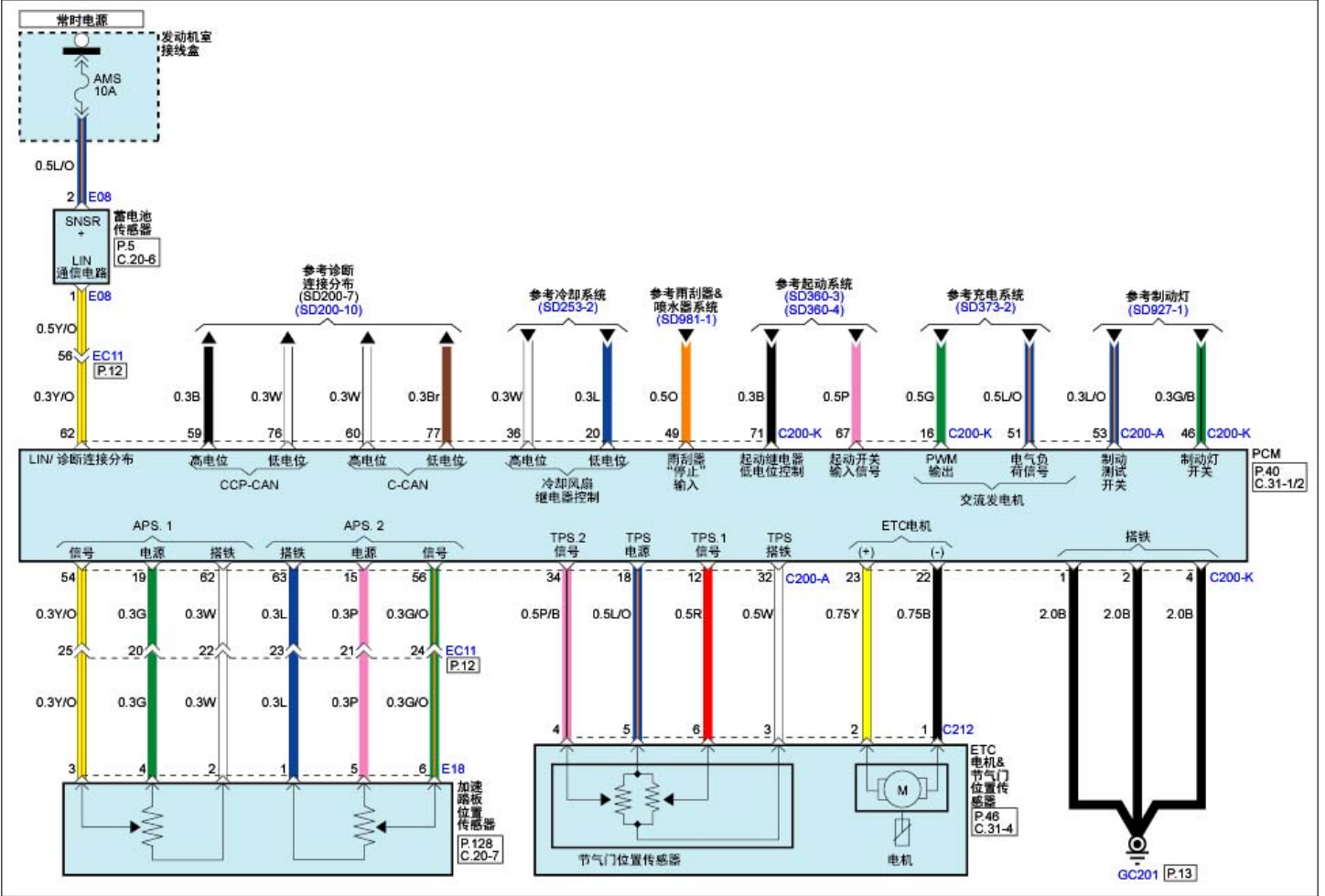
发动机控制系统(G4NA : NU 2.0L MPI)(6)
